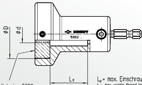
Gewinde-Gutlehring 5382 GO screw ring gauge 5382
