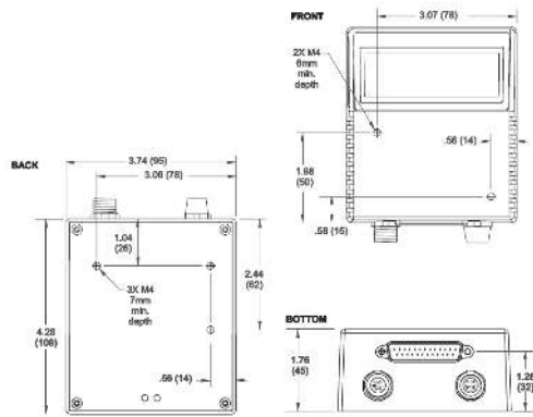
MS-860 Dimensions
