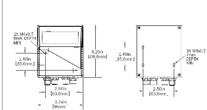
QX-870 Dimensions
